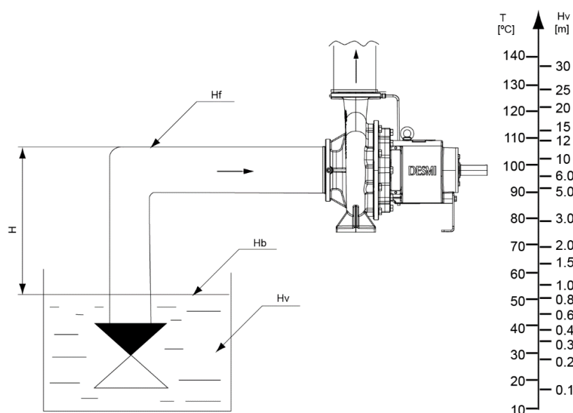
图5-6：吸上高度
