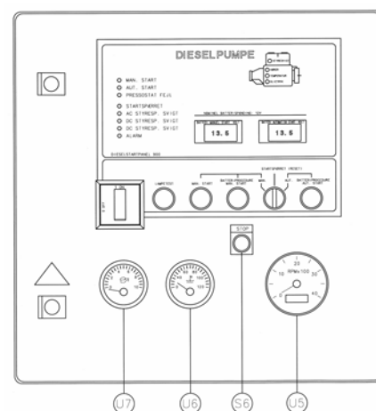
Figur 3: Styretavle (diesel)
