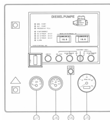
Figur 3: Styretavle (diesel)
