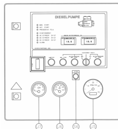
Figur 3: Styretavle (diesel)
