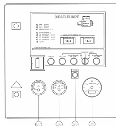
Figur 3: Styretavle (diesel)
