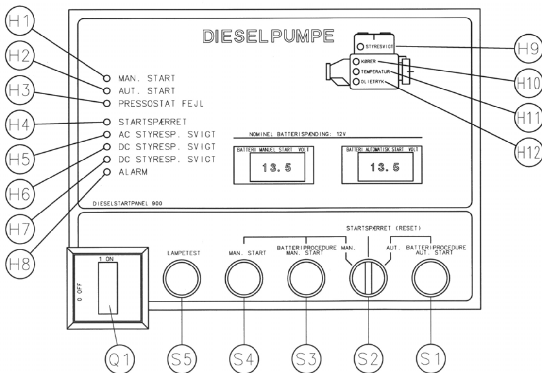
Figur 2: Lamper, indikeringer og omskifter
