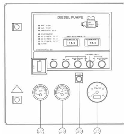
Figur 3: Styretavle (diesel)
