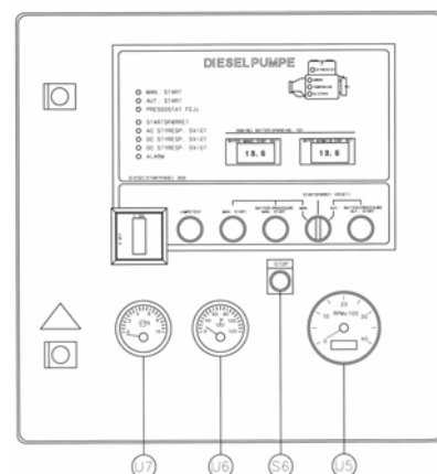
Figur 3: Styretavle (diesel)
